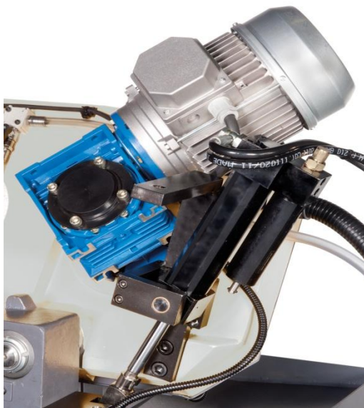
DETALLE BAJADA HIDRAULICA
